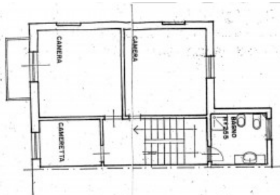
PIANO PRIMO h. 350
